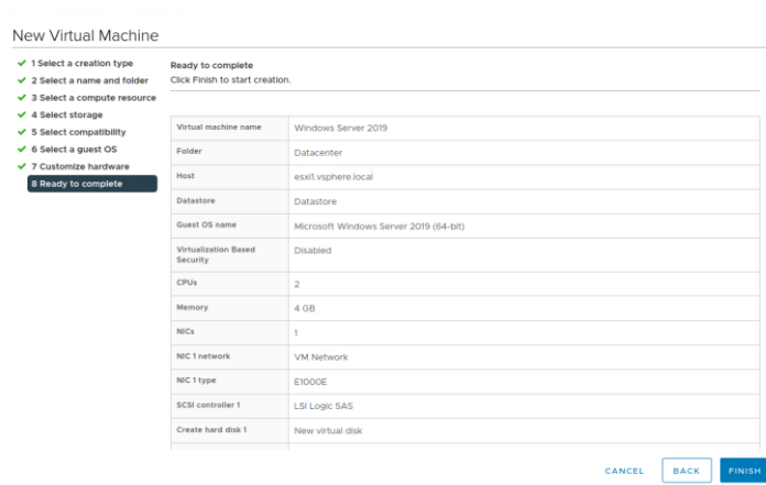
Slika 6.9 Sumarizirani prikaz postavki virtualne mašine
