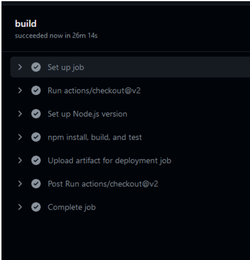
Slika 4.16 Izgradnja aplikacije
