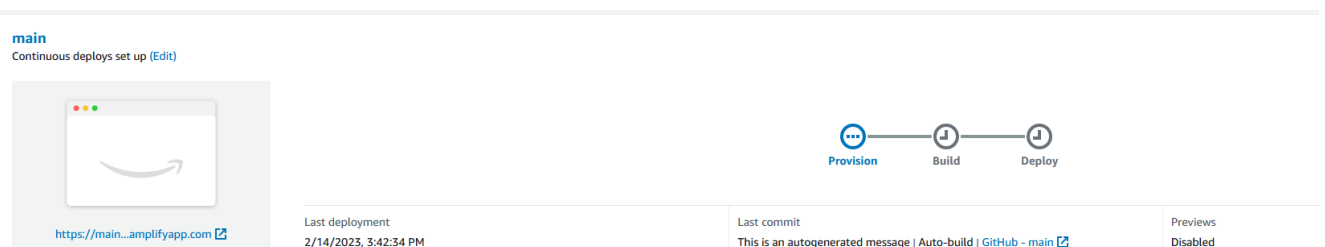
Slika 4.8 Proces razvoja
