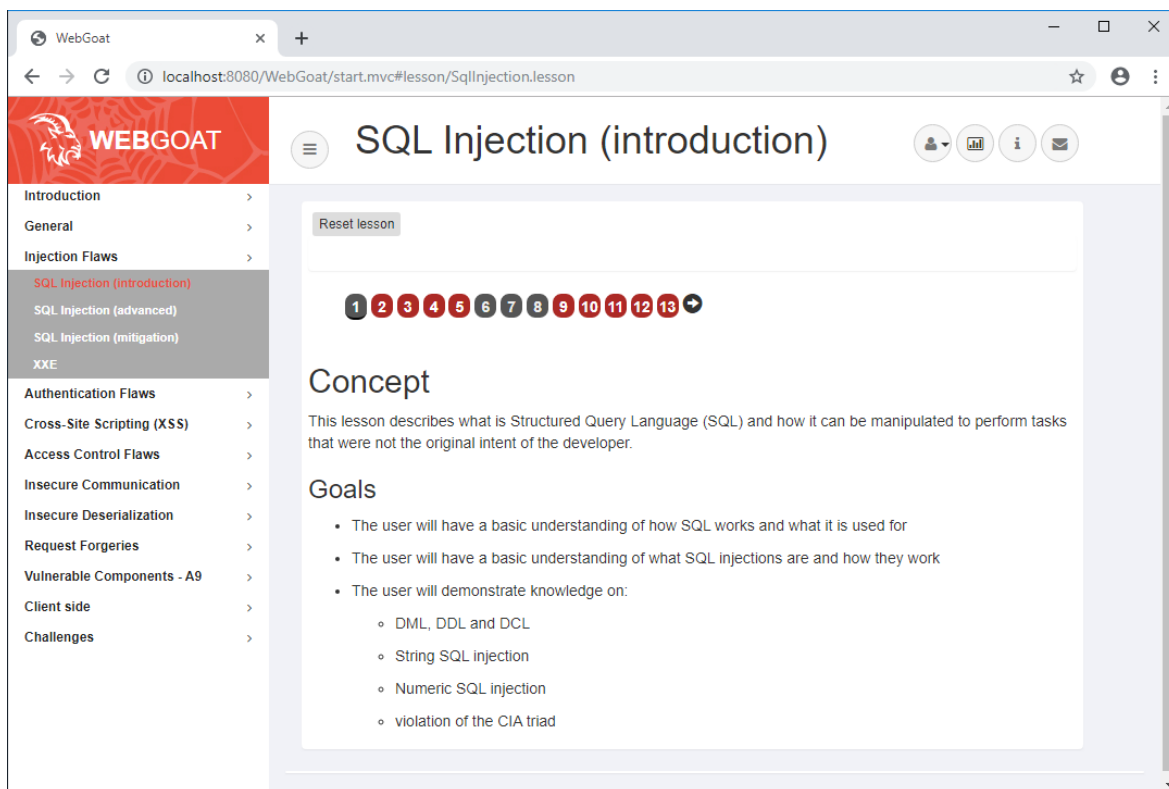
Slika 5.1 WebGoat aplikacija
