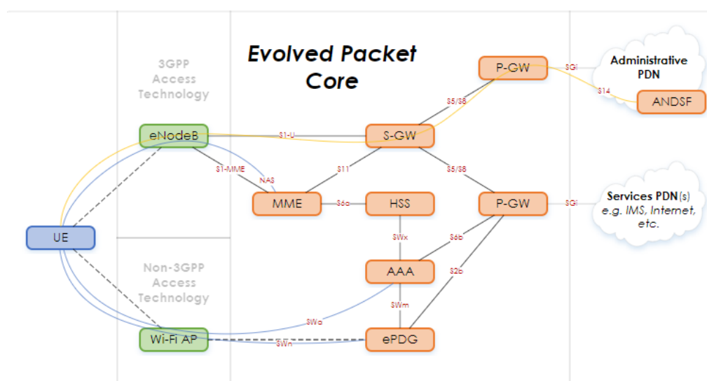
Slika 2.4.13 Evolved Packet Core, jezgra mreže LTE [7]
