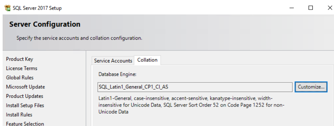
Slika 5.5 SQL collation
