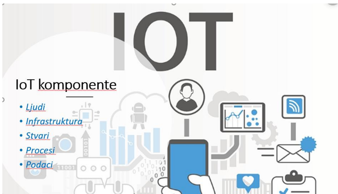
Slika 2-1 IoT komponente
