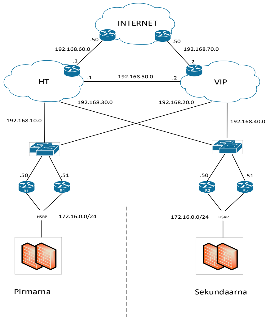
Slika 9.1 Shematski prikaz javne mreže 36
