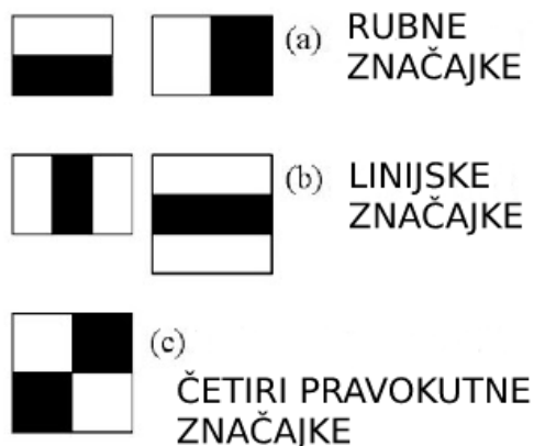
Slika 22. Prikaz haar značajke[22]
