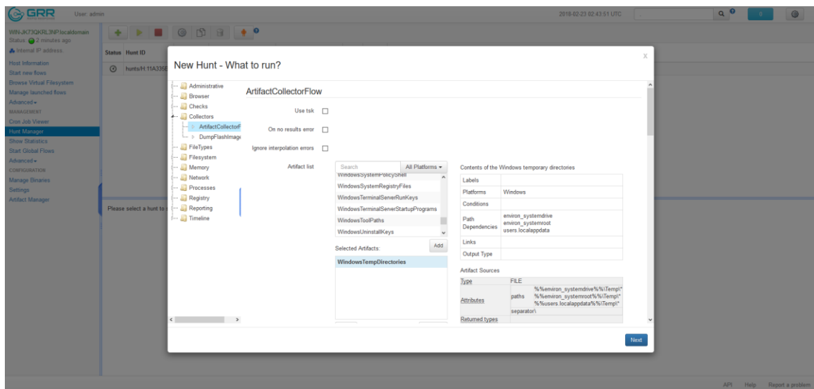
Slika 3.5 Odabir artefakta "WindowsTempDirectories"
