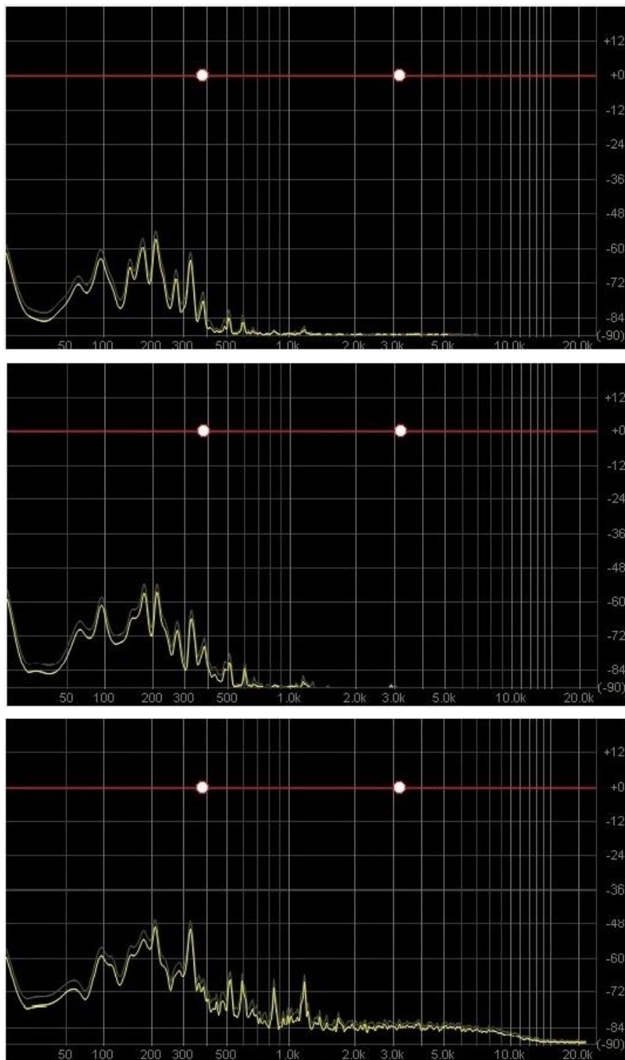
Slika 4.1. Usporedba valnog signala tri miksana zvuka – originalnog bez efekata, miksa baziranog na CUDA softverskom plugin-u i miksa baziranog na hardverskom uređaju kojeg CUDA softverski plugin emulira
