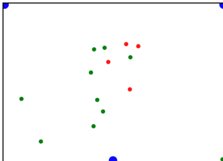
Slika 5.3 - Prikaz mjerenja pozicije radiofarova u Testu 1 sa konstantom za okoliš 2
