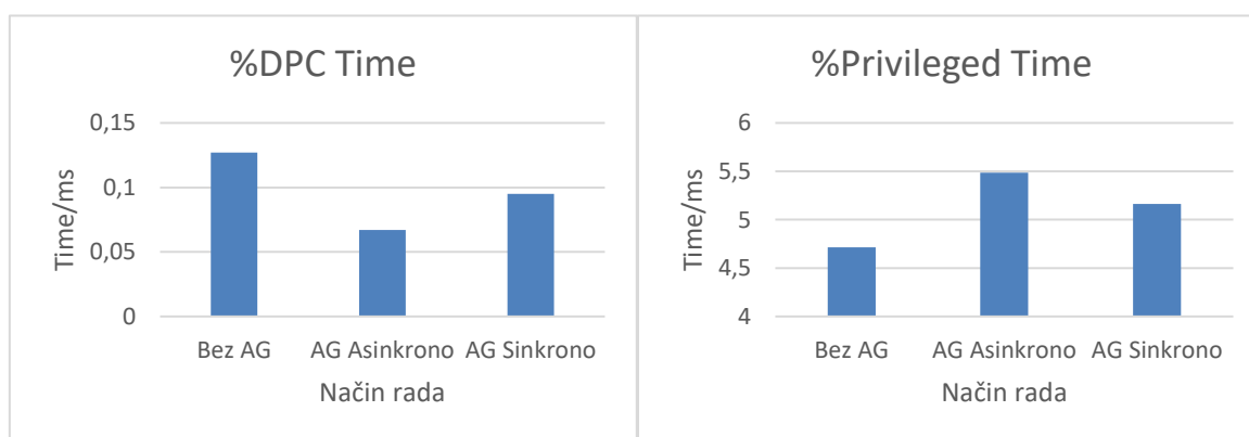
Slika 7.6 Brojači performansi iz kategorije " Processor "
