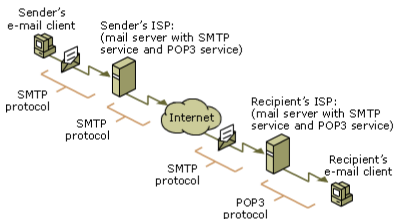
Slika 1. SMTP protokol
