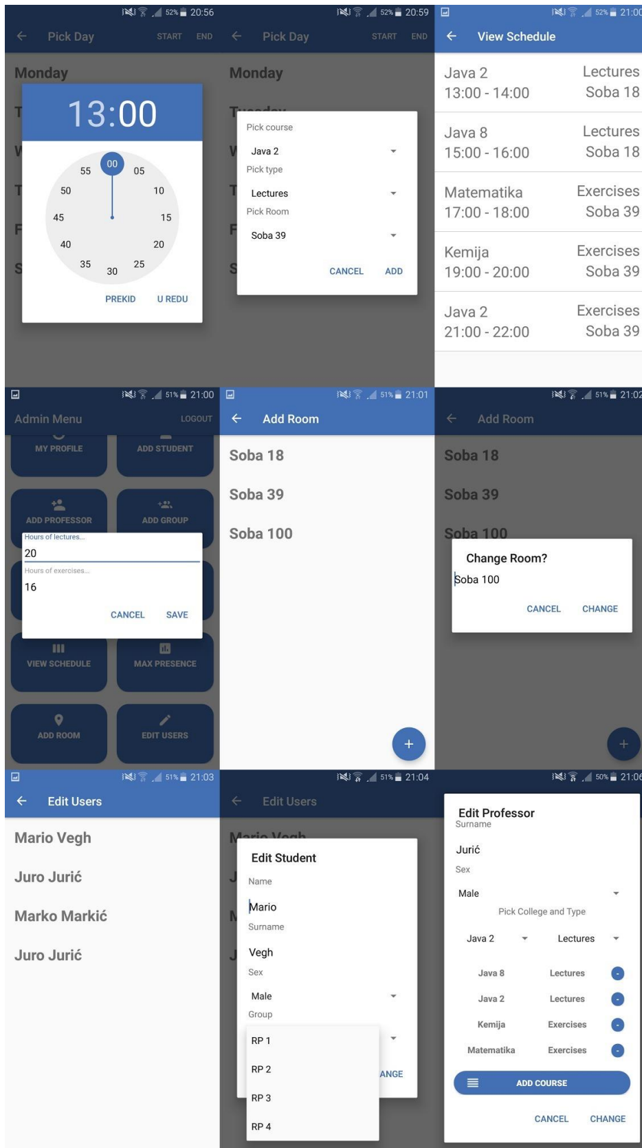
Slika 42. Sučelje role administrator (2)
