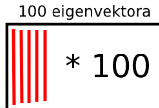
Slika 32. Prikaz kovarijance matrice u nižoj dimenziji
