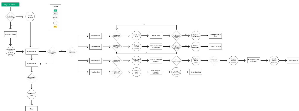
Slika 3 FlowChart aplikacije
