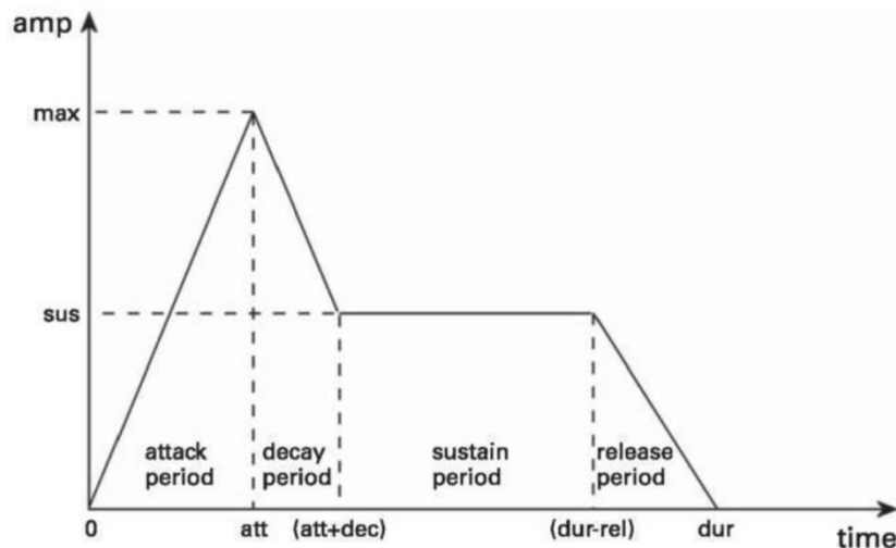
Slika 7 Zvučna omotnica 10
