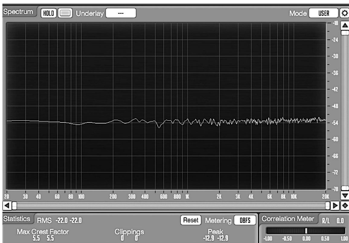
Slika 12 Bijeli šum
