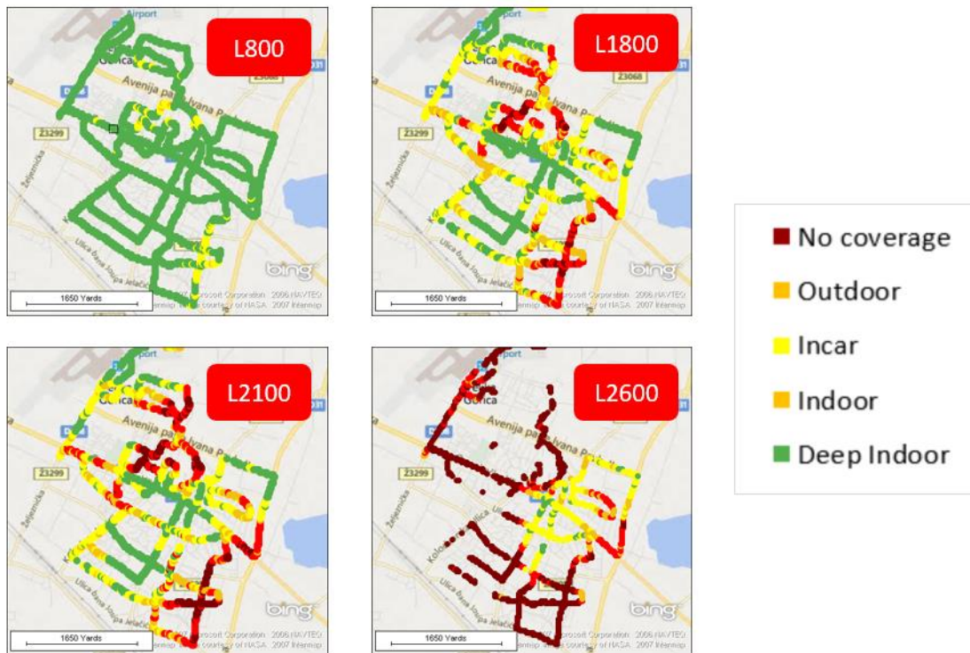
Slika 4.5.7 Frekvencijski pojasi korišteni u Velikoj Gorici za A1
