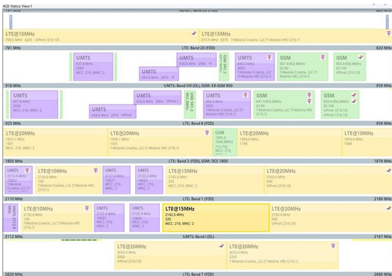
Slika 2.4.14 Frekvencijski pojasevi po tehnologijama i operaterima
