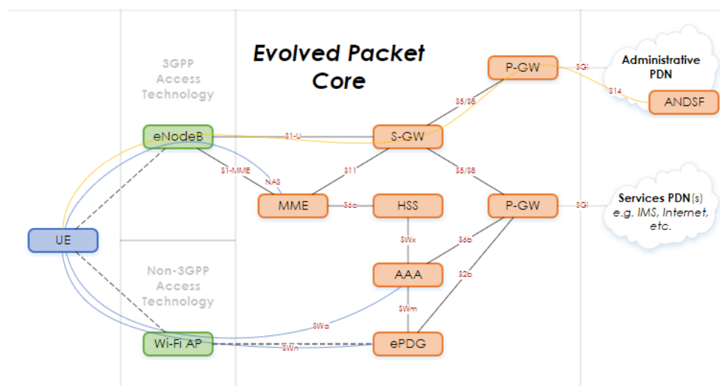
Slika 2.4.13 Evolved Packet Core, jezgra mreže LTE [7]
