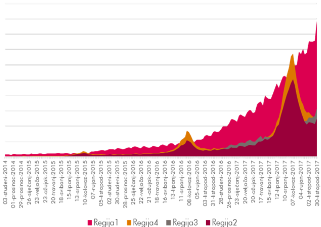
Slika 2.4.11 LTE podatkovni promet za razdoblje 2014. - 2017.
