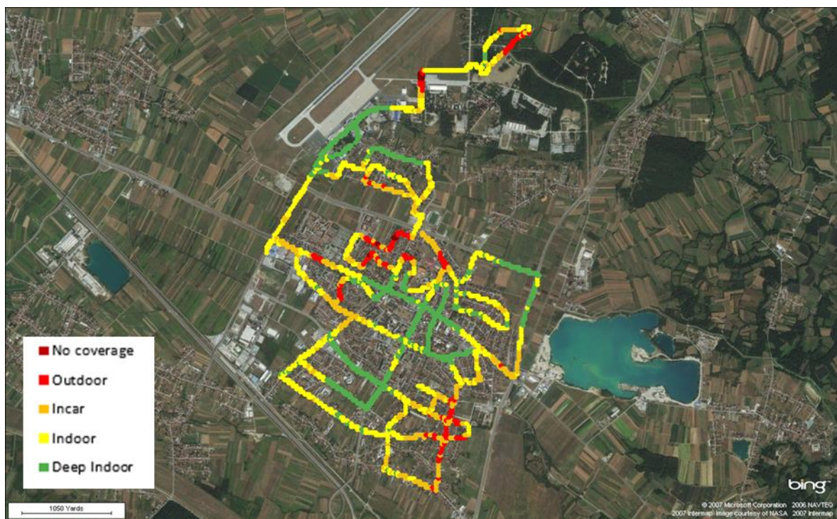
Slika 4.1.1 Jakost LTE signala RSRP na području grada Velika Gorica
