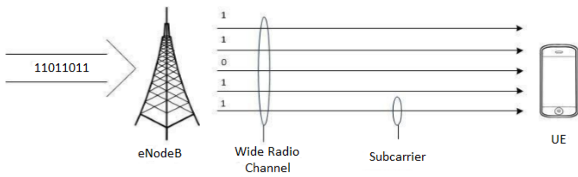
Slika 2.4.1 OFDMA [10]
