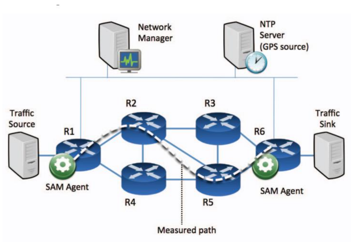
Slika 2.4.21 Aktivno mrežno mjerenje [16]
