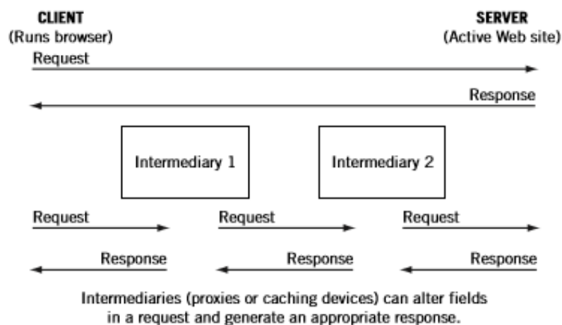
Slika 4.4.2 HTTP interakcija [23]
