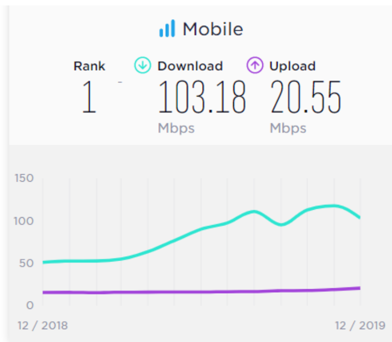
Slika 3.2.2.2 Prosječna download i upload brzina Južne Koreje [21]
