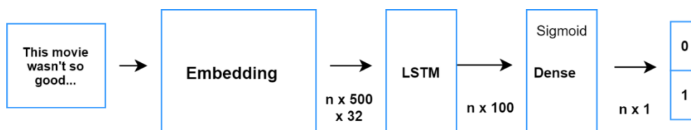
Slika 9. LSTM neuronska mreža
