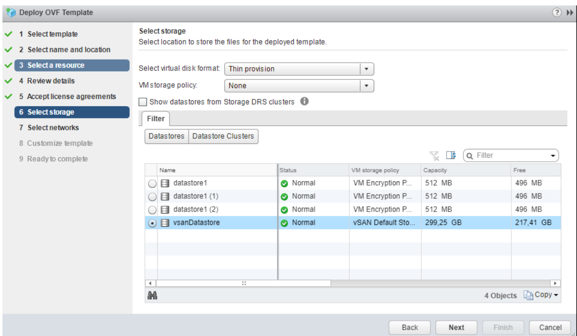
Slika 3.5 Odabir datastore-a
