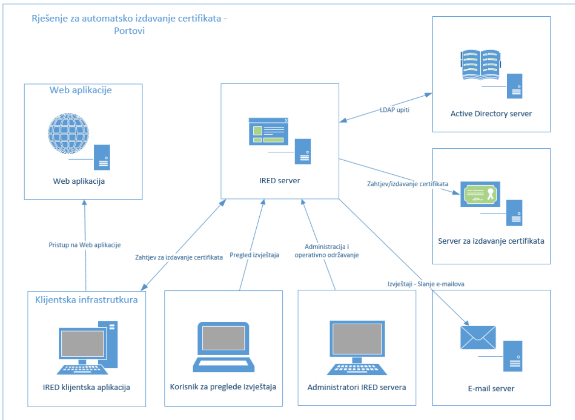
Slika 4.9 Port zahtjevi
