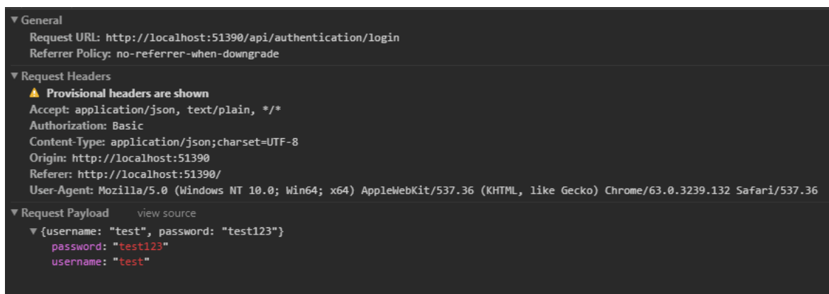
Slika 5.12 Login - zahtjev
